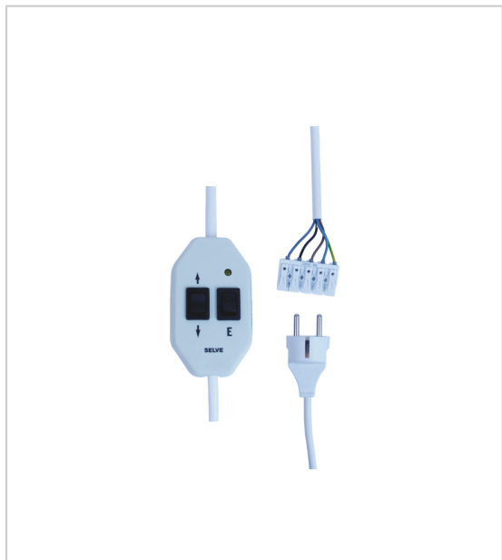
Câble de réglage à 5 fils pour moteurs SELVE SE ET SE-RC
