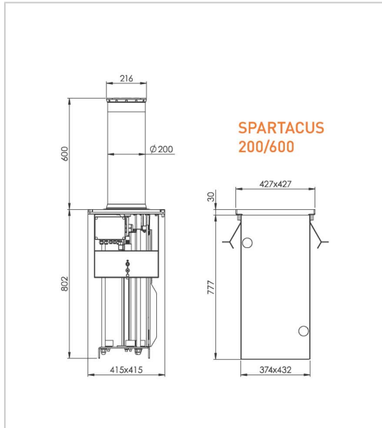
Caisson de fondation pour borne escamotable SPARTACUS
