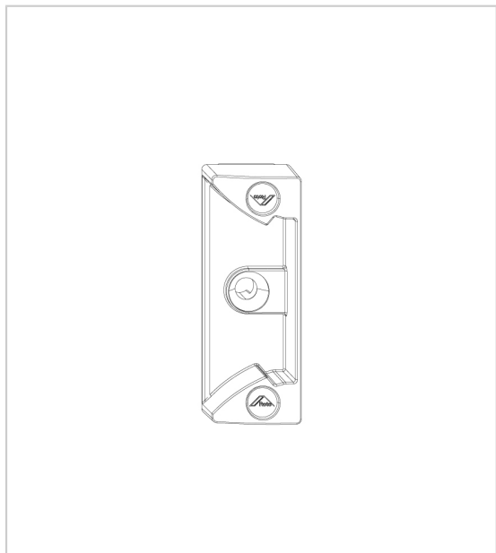
Gâche pour loqueteau mécanique ROTO NX
