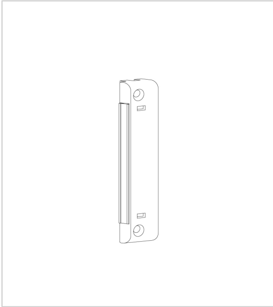
Loqueteau magnétique ROTO NT sur dormant PVC
